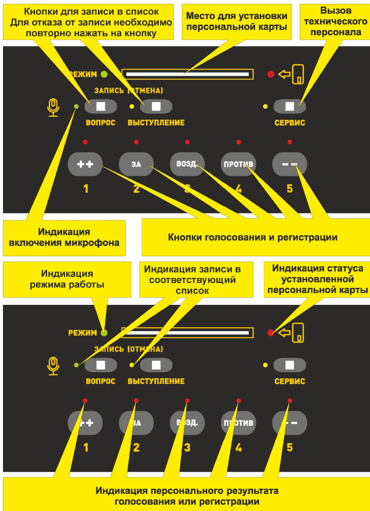
Рисунок 2. Назначение элементов управления и индикации индивидуального пульта
